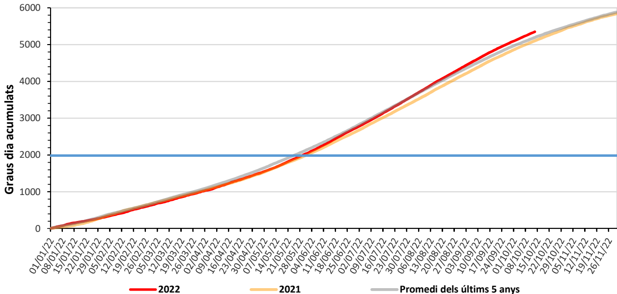
Graus dia acumulats Castelló Sud - València Nord
