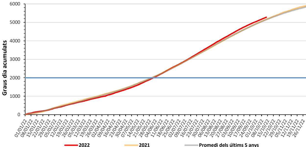
Graus dia acumulats València Interior
