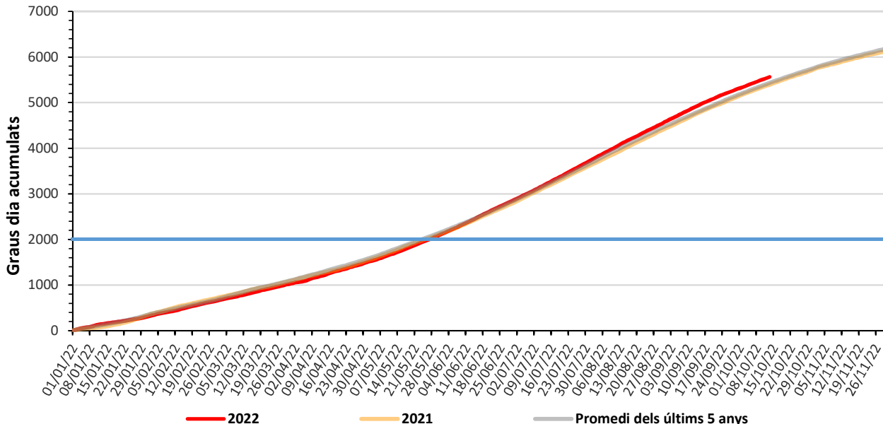
Graus dia acumulats València Sud - Alacant Nord
