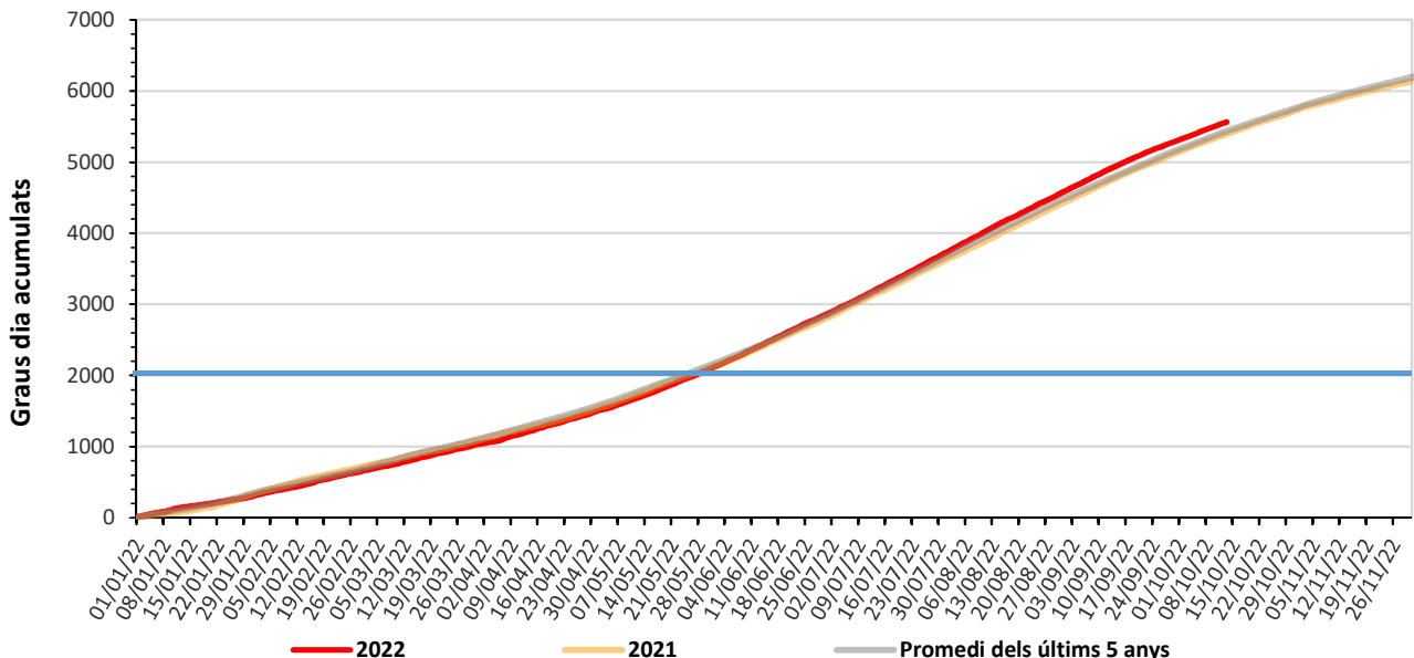
Graus dia acumulats Alacant Sud
